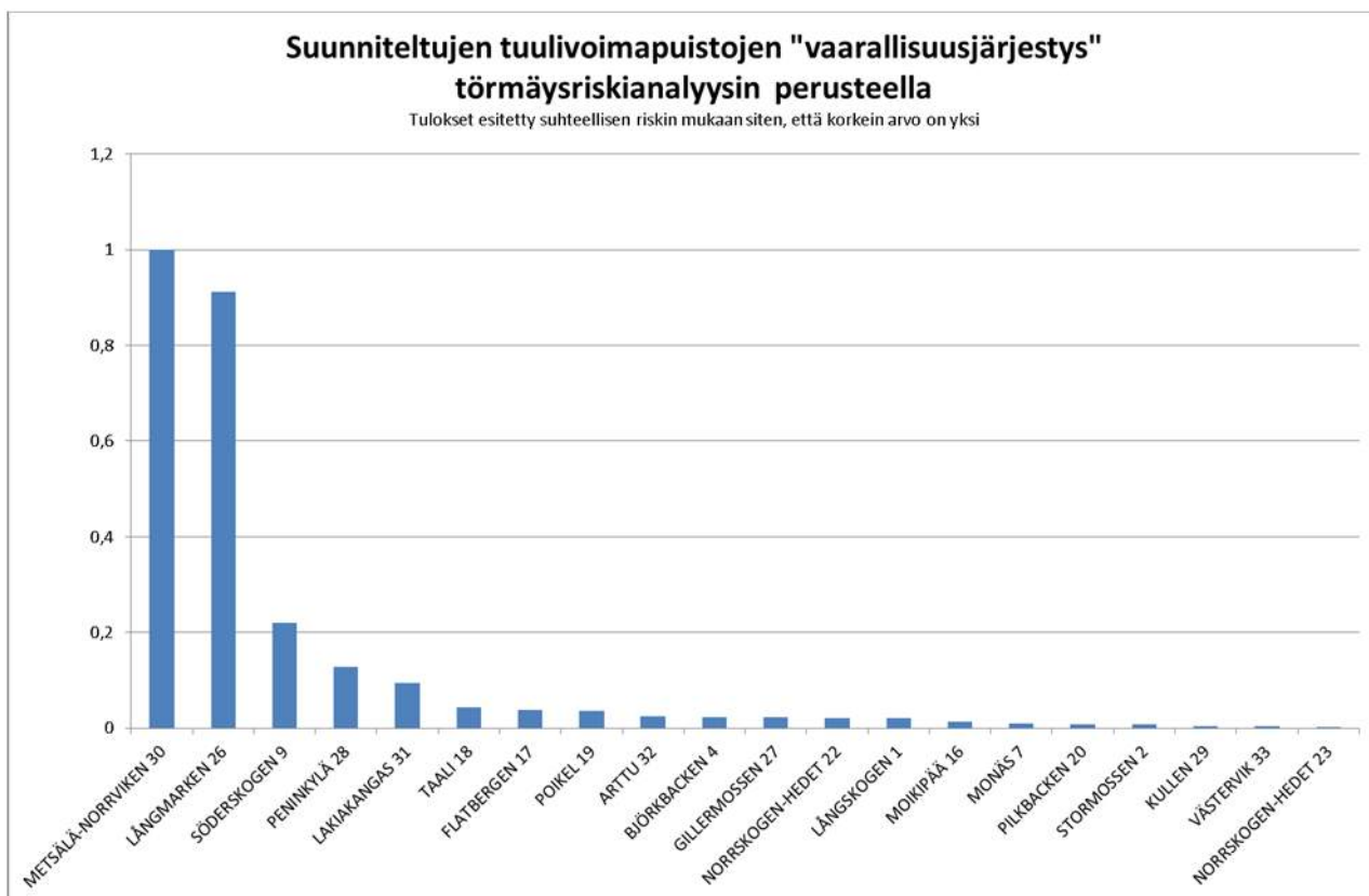
Kuva 29. Tuulivoima-alueiden sääksen kohdistama törmäysriski pesimäaikana
