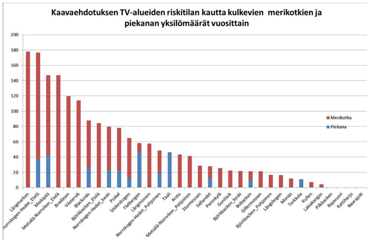
Kuva 22. Muuttavien merikotkan ja piekanan törmäysriskin tarkastelua TV-alueittain.
