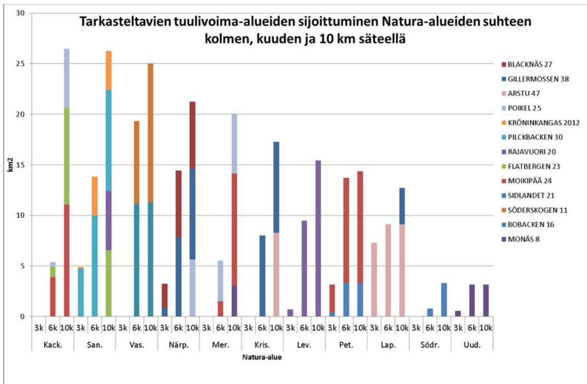
Kuva 31. TV-alueiden sijoittuminen Natura-alueisiin nähden
