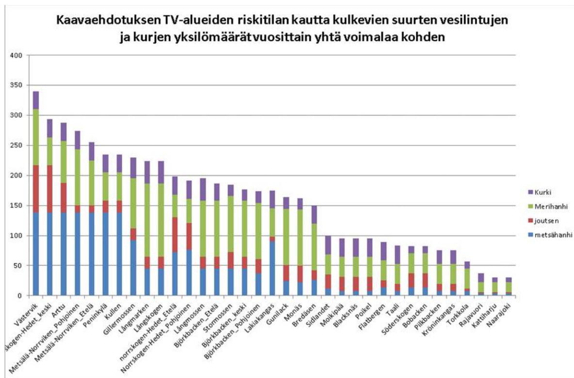
Kuva 23. Kaavaehdotuksen tv-alueiden riskitilan kautta lentävien lintujen yksilömäärät yhtä voimalaa kohden.
